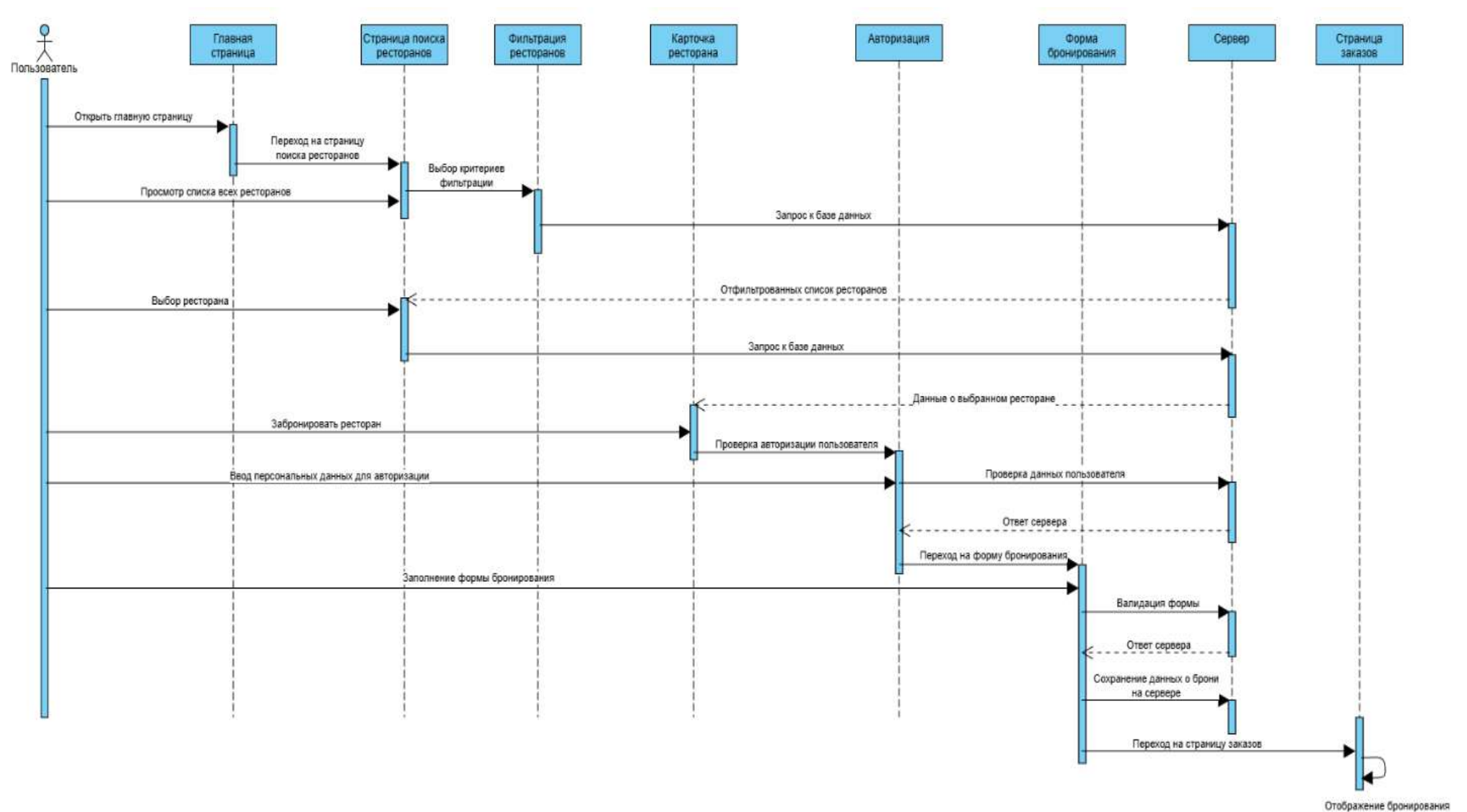
Рисунок 2 – Диаграмма последовательности
