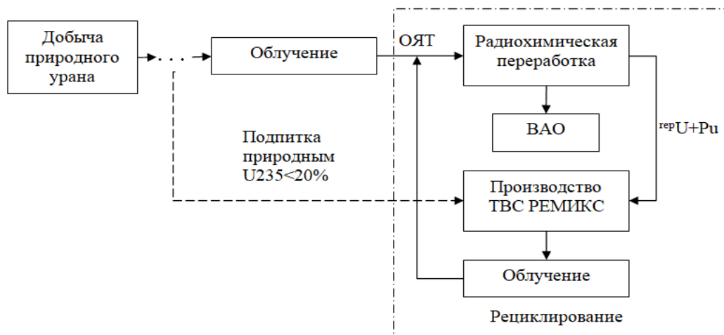
Рисунок 2 – Схема рециклирования РЕМИКС-А при обогащении подпитки до 20% по U235, где ВАО – высокоактивные отходы; ТВС – тепловыделяющая сборка; ^{238}\text{U} – регенерированный уран.
