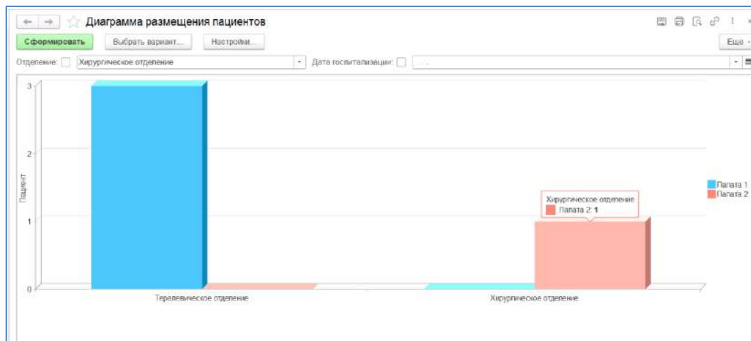
Рисунок 9 – Отчет «ДиаграммаРазмещенияПациентов»
