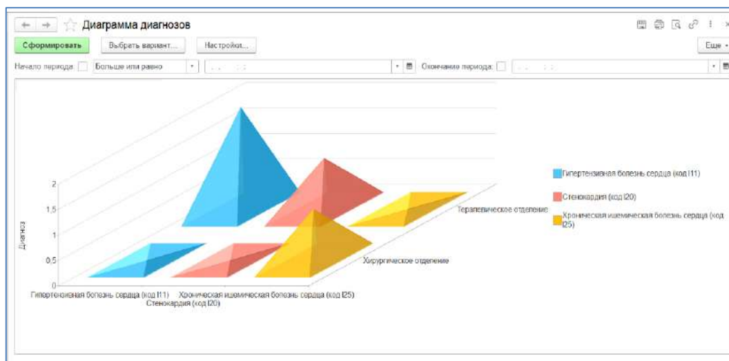
Рисунок 10 – Отчет «ДиаграммаДиагнозов»
