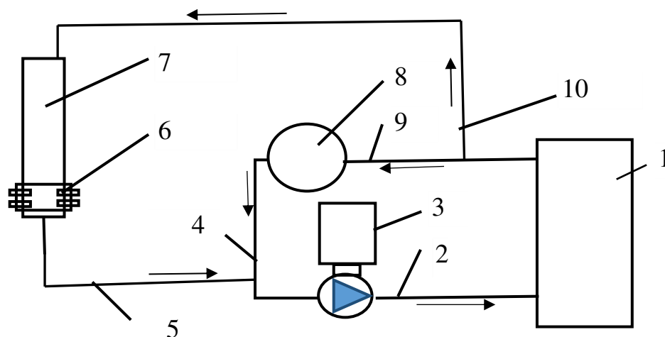
Рисунок 2 – Предлагаемая схема включения компенсатора давления в первый контур системы циркуляции двухконтурной ядерной энергетической установки:
