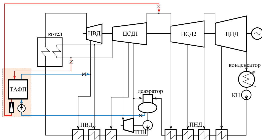
Рисунок 1 – Принципиальная схема паротурбинной установки с аккумуляцией теплоты перегретого пара в ТАФП
