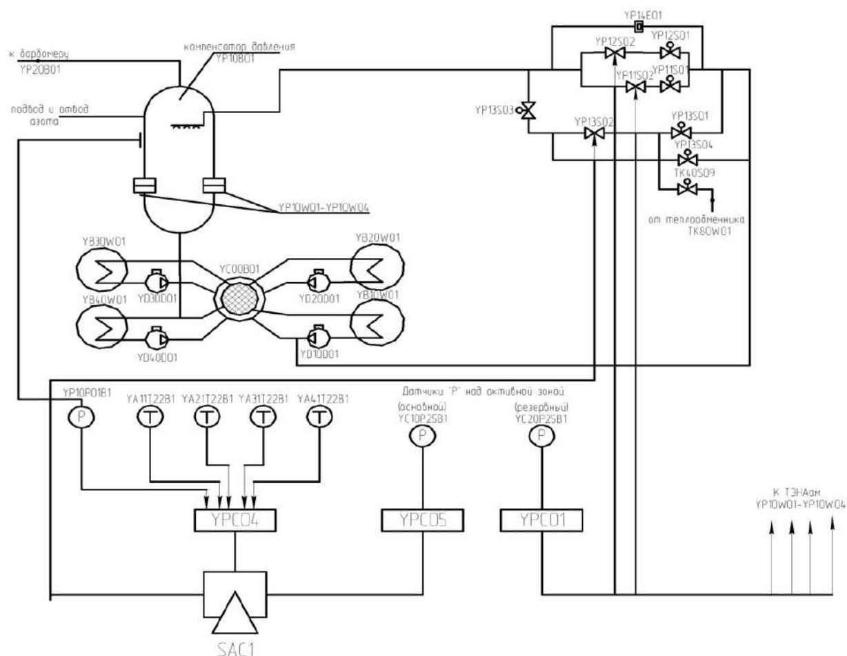
Рисунок 1 – Схема САУ давления и разности температур
